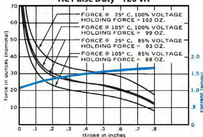
AC Pulse Duty - 120 VA
