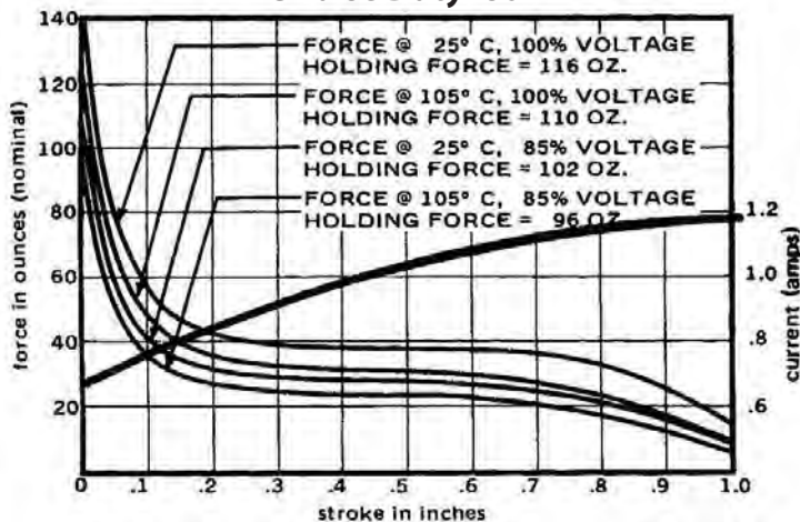
AC Pulse Duty - 80 VA
