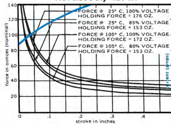
AC Pulse Duty- 120 VA
